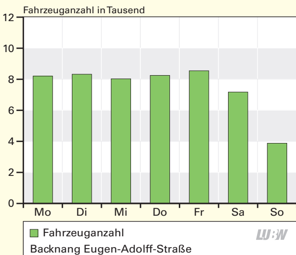
Mittlerer Wochengang der Gesamtverkehrsstärke, Stickstoffdioxid- und Partikel PM 10 -Konzentration an der Verkehrszählstelle Backnang Eugen-Adolff-Straße 2020; Basis: Tagesmittelwerte
