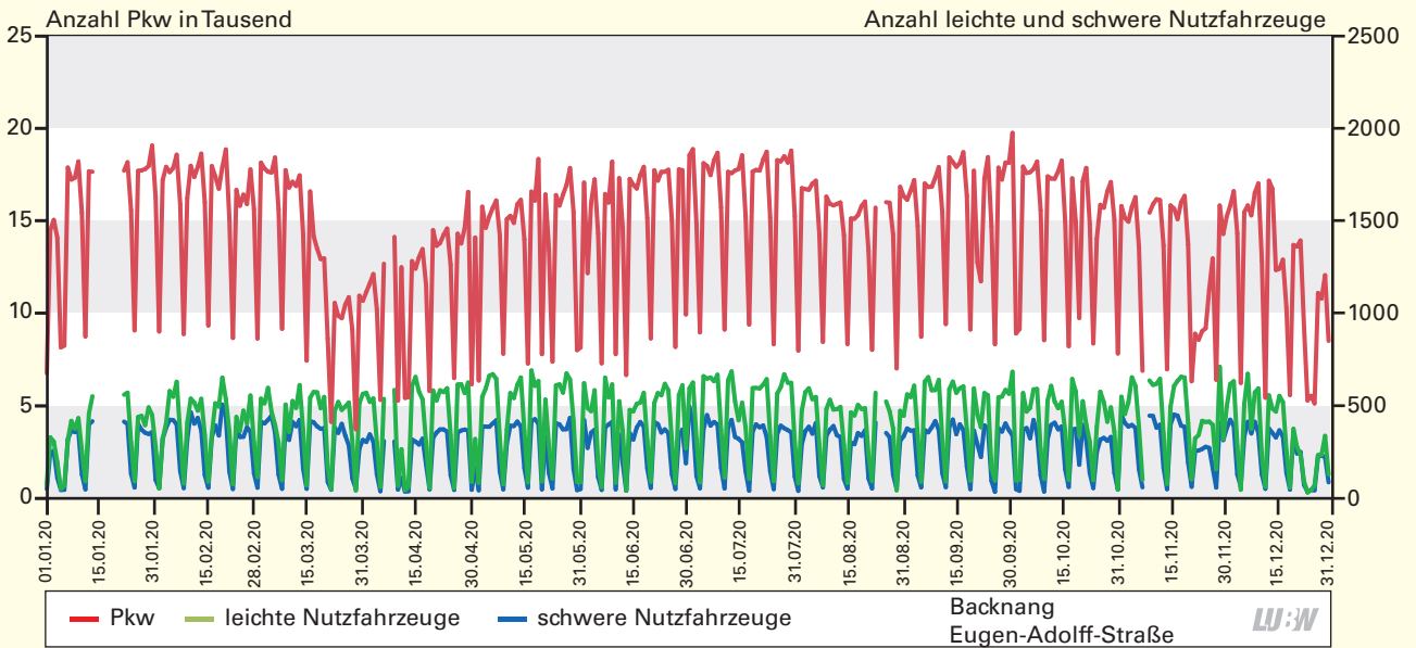
Verlauf der täglichen Verkehrsstärken der 3 Fahrzeugklassen am Standort Backnang Eugen-Adolff-Straße 2020
