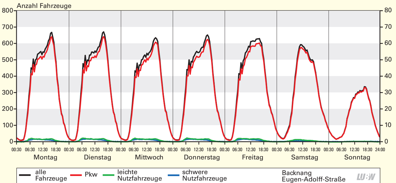
Mittlerer Wochengang der Verkehrsstärken der 3 Fahrzeugklassen sowie der Stickstoffdioxidkonzentration an der Verkehrszählstelle Backnang Eugen-Adolff-Straße 2020; Basis: Halbstundenwerte
